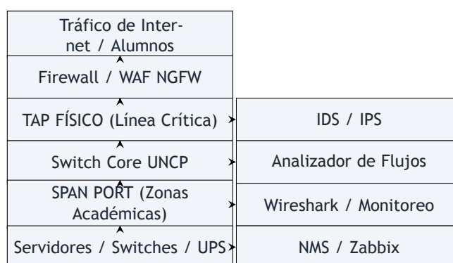
Figura 3: Arquitectura de telemetría de red UNCP - Fase I
